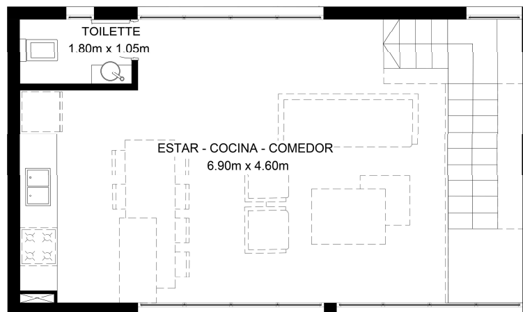
PLANTA ALTA
