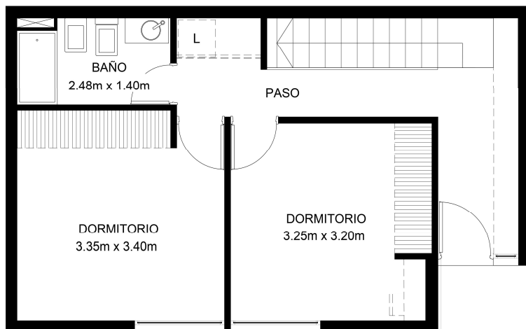
PLANTA BAJA
