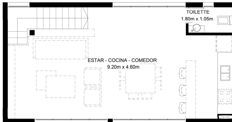
PLANTA ALTA
