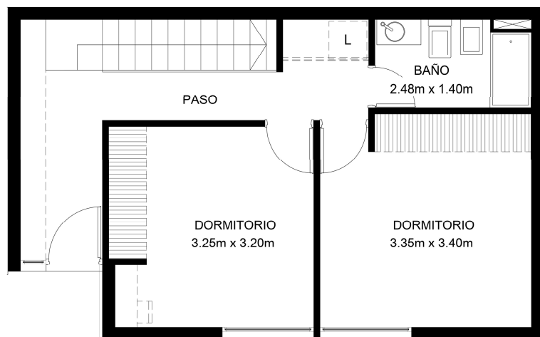
PLANTA BAJA
