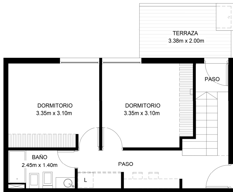
PLANTA BAJA
